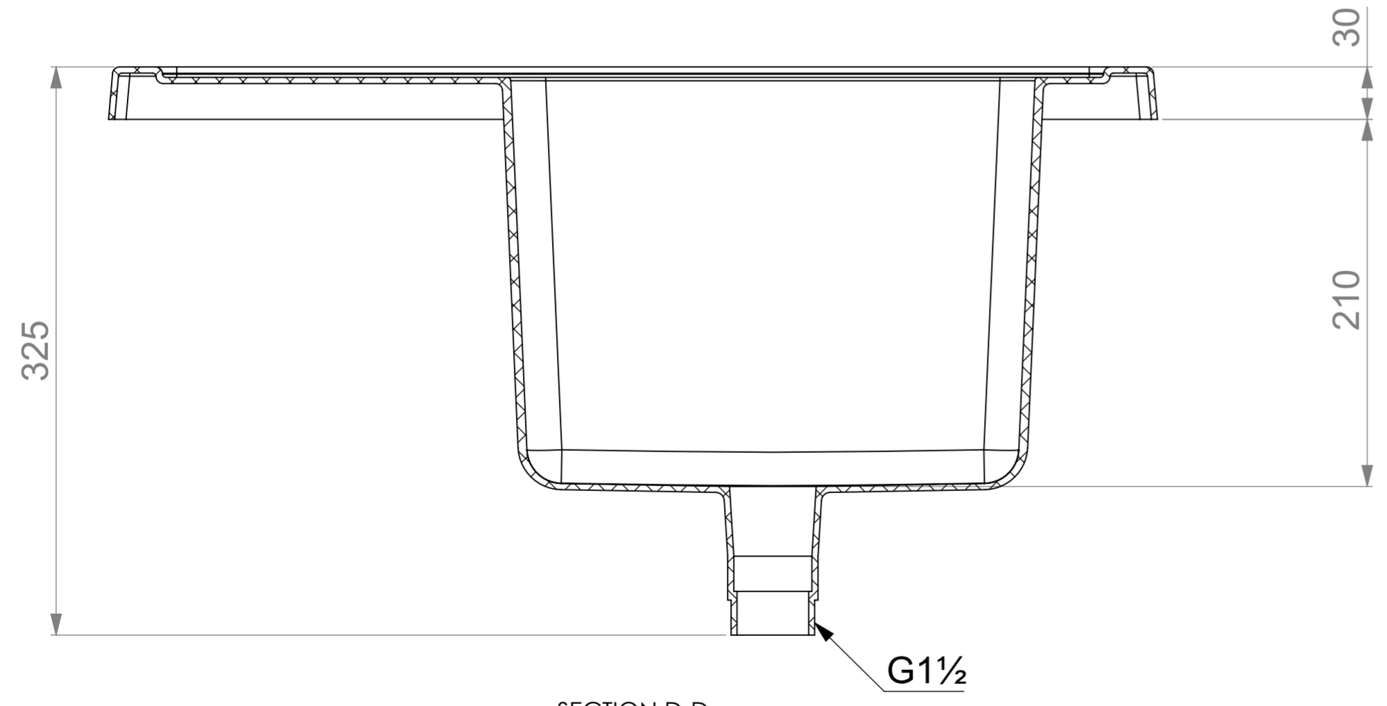
SECTION D-D
